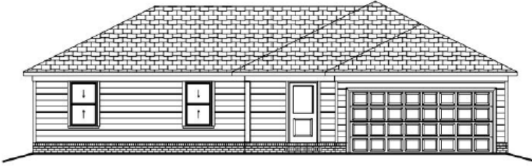
Elevation A
